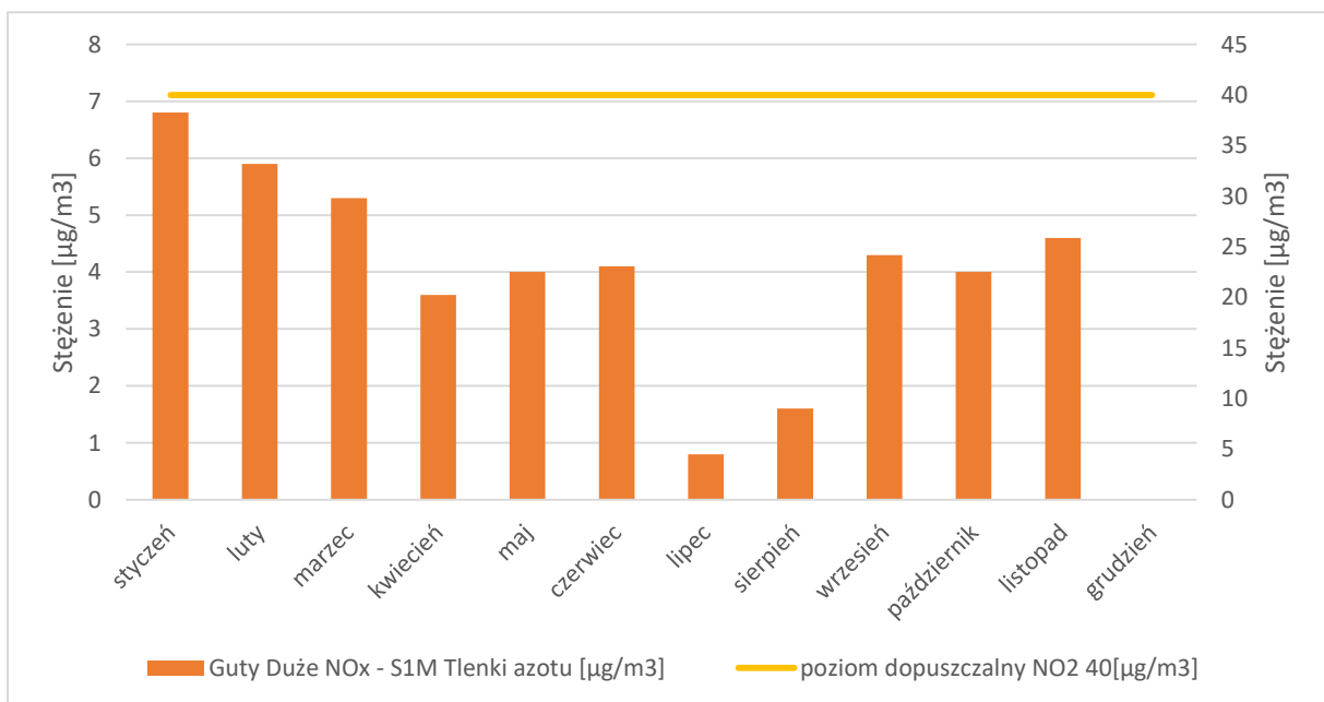
Ryc. 8. Stężenie średniodobowe dwutlenku azotu NO 2 w ujęciu miesięcznym w 2018 roku
