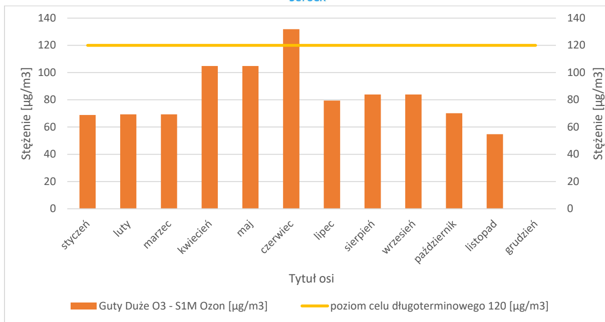
Ryc. 9. Stężenie ozonu w poszczególnych miesiącach roku 2018
