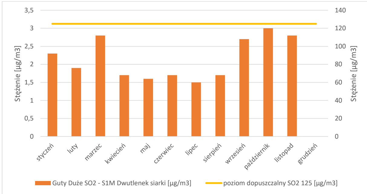
Ryc. 7. Stężenie średniodobowe dwutlenku węgla SO 2 w ujęciu miesięcznym w 2018 roku
